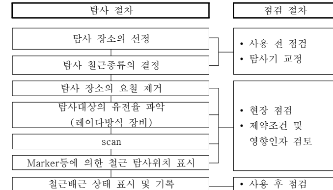
[그림 16] 철근탐사 및 장비 점검 등의 절차
