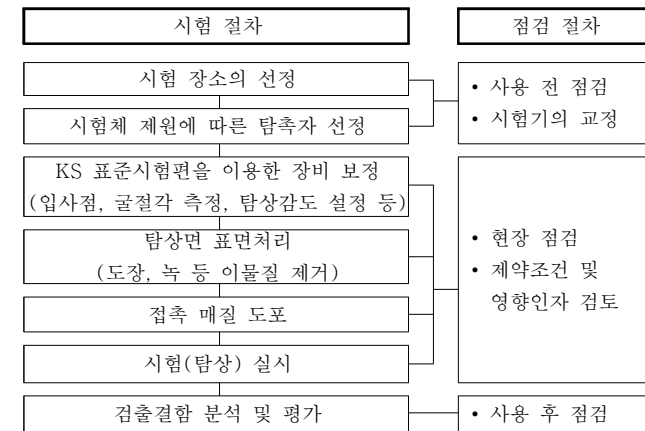
【그림 22】 강재 초음파시험 및 탐상기 점검 등의 절차
