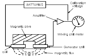
[그림 14] 전자기유도 방식에 의한 철근탐사장비의 구성
